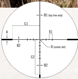
VMR-2 MOA
